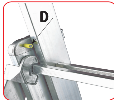
Dispositivo anti-ribaltamento del terzo tronco (Luxe3) Impedisce che il terzo tronco sfugga di mano e cada mentre lo si sfilava in posizione a cavalletto.
